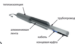
Установка на трубе
